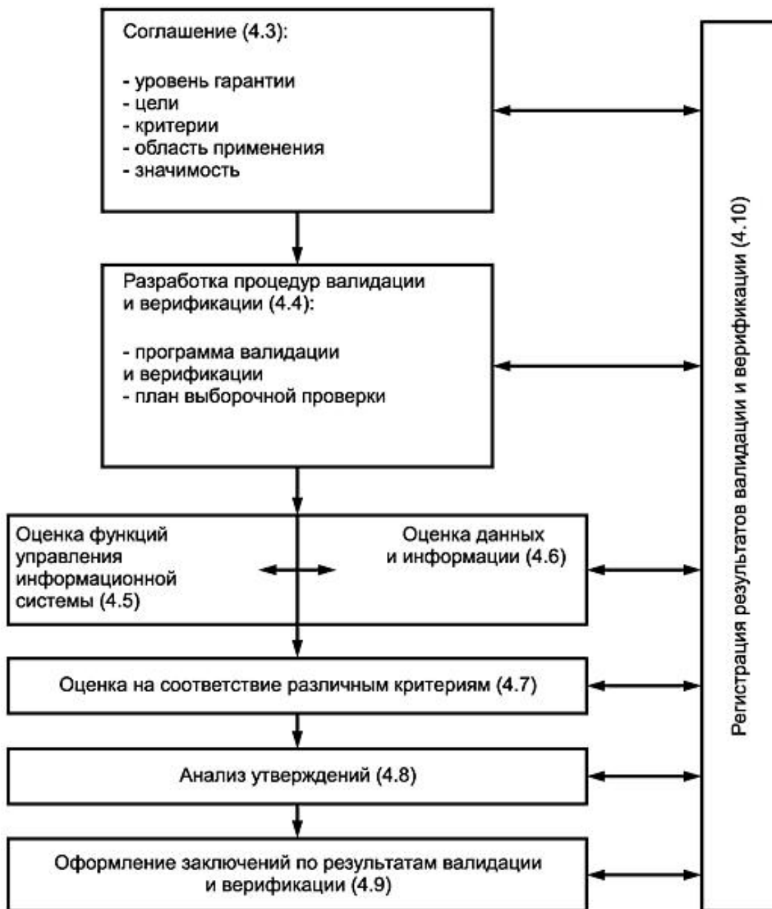
Рисунок 2 - Процесс валидации и верификации
